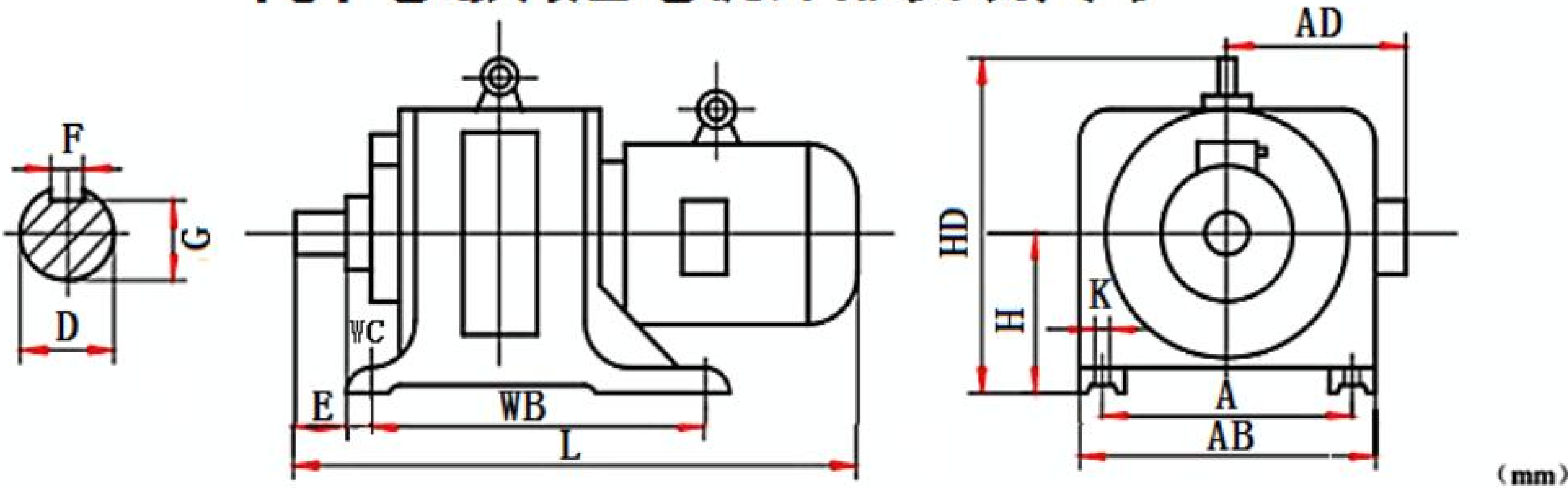
YCT电磁调速电机外形安装尺寸
