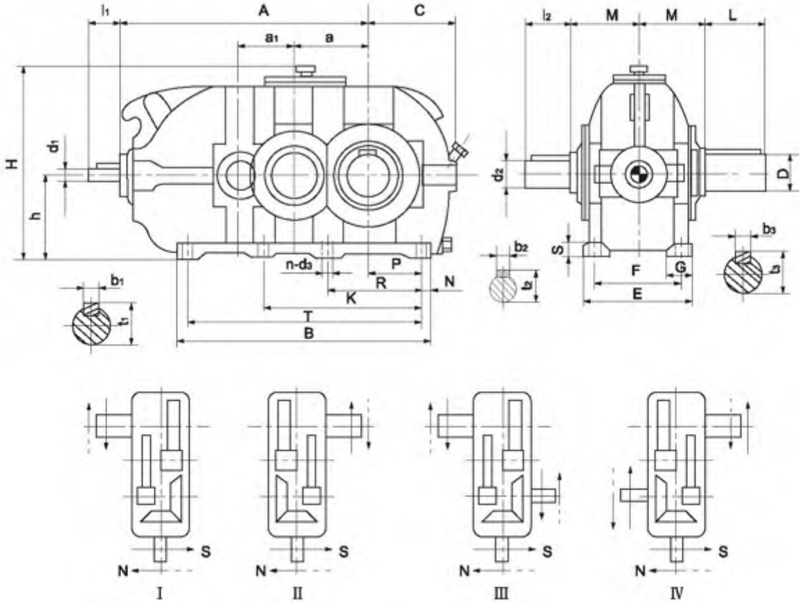
DCY、DCZ型装配型式
