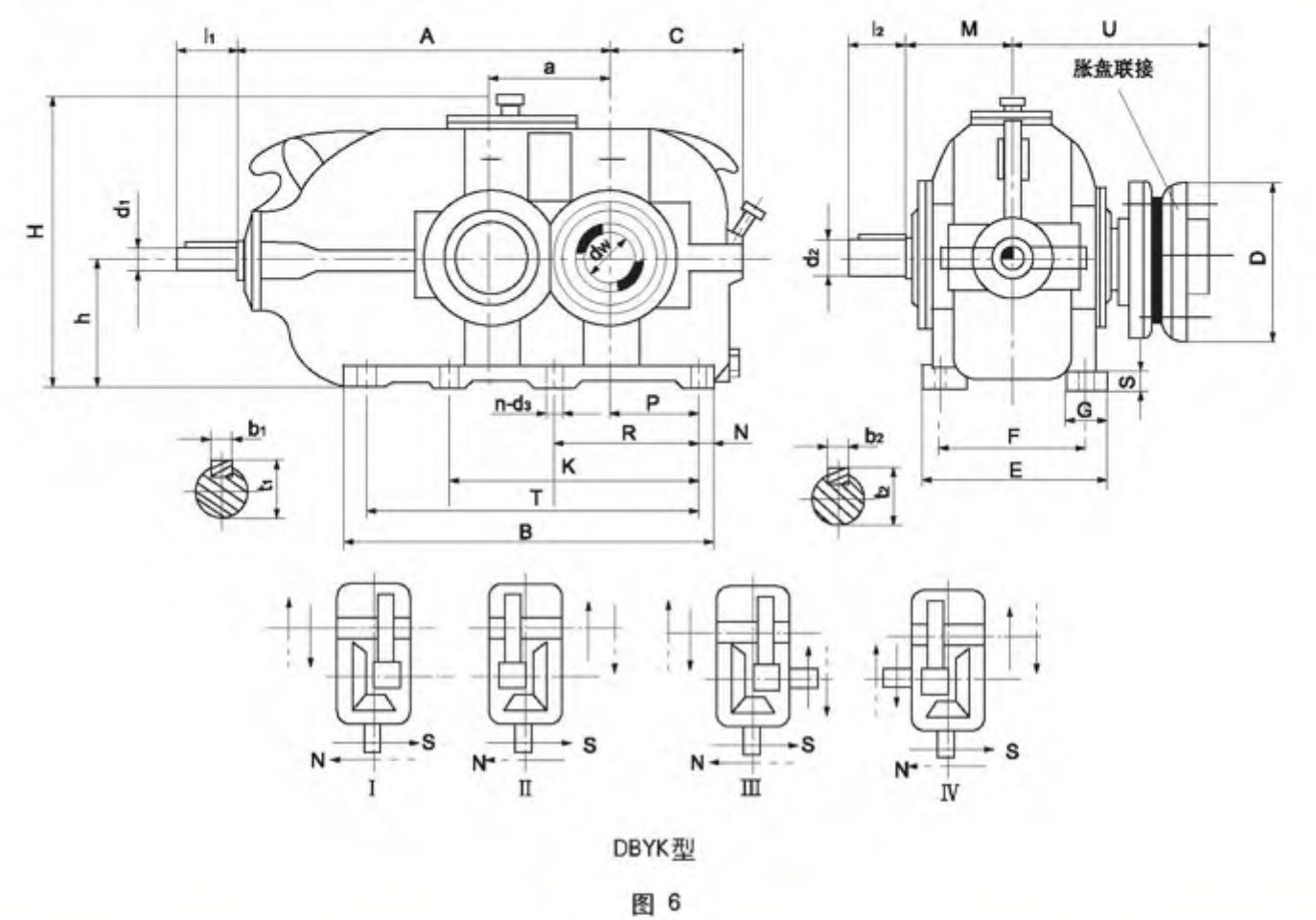
6、DBYK减速器的装配型式及外形尺寸见图6，表26
