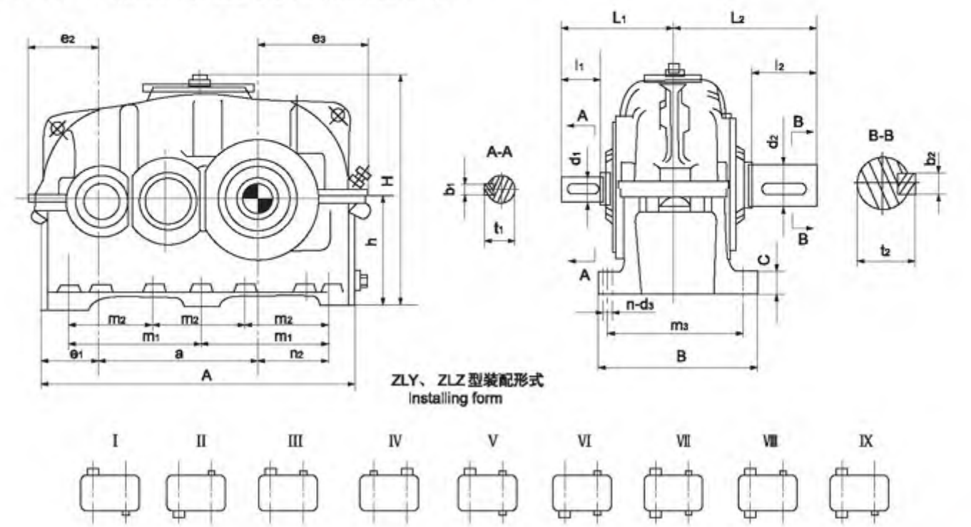
2、ZLY, ZLZ减速器的装配型式及外形尺寸见图2, 表22
