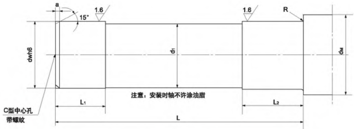
图 10 胀盘联接的轴
