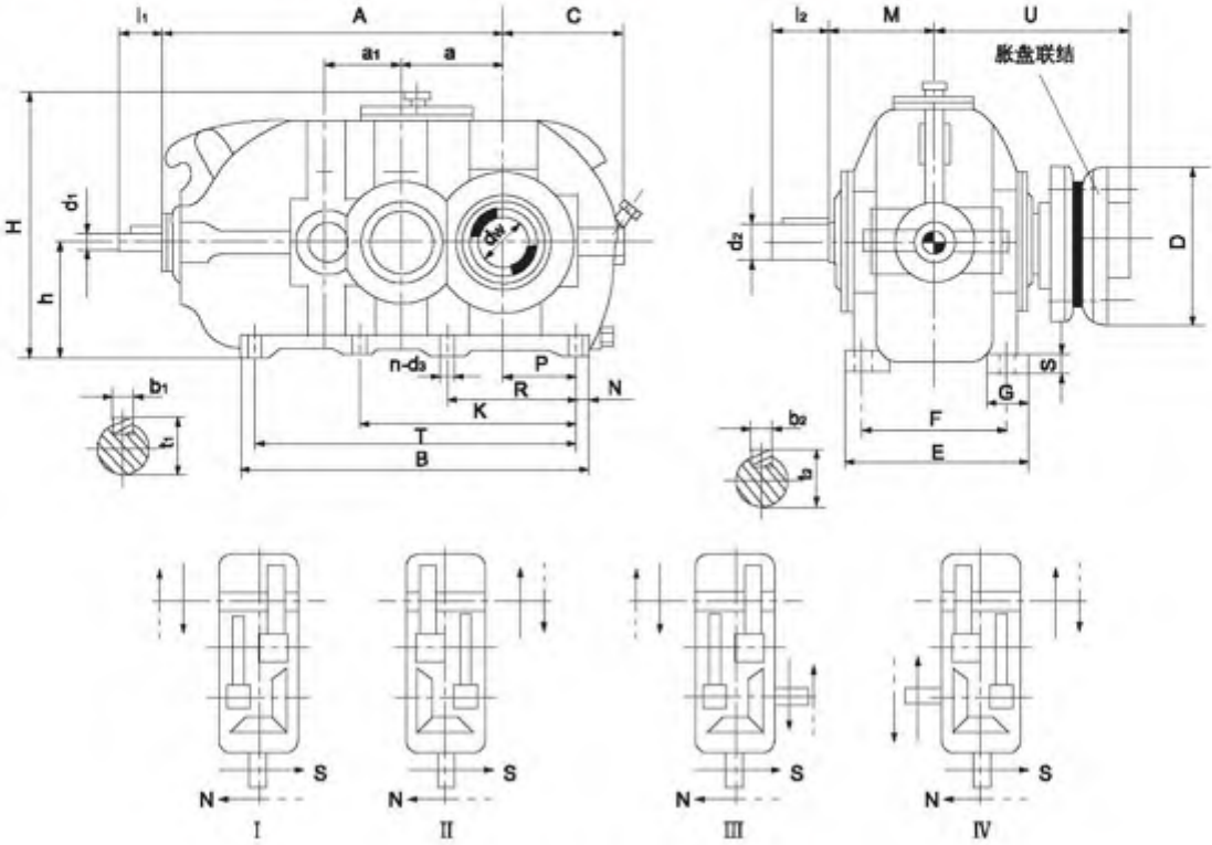
DCYK型装配型式
