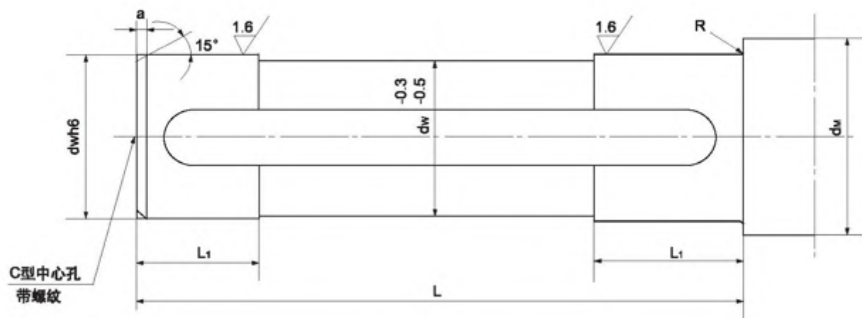
图 11 平键联接的轴
