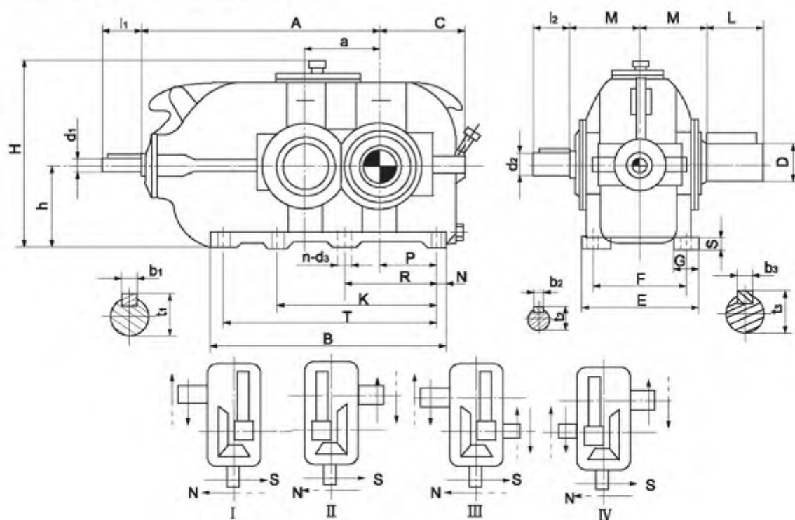
DBY、DBZ型装配型式
