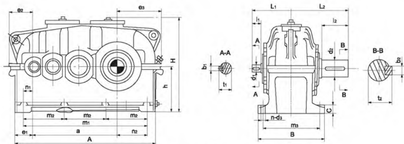
ZSY、ZSZ 型装配型式
