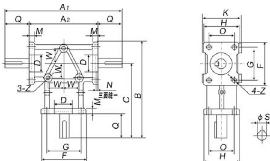
ARA 系列外型尺寸图:
