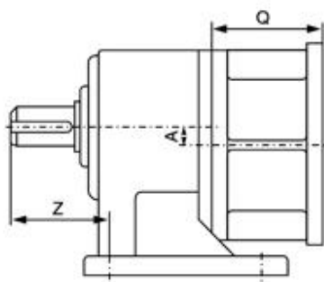
GL(H)WK
