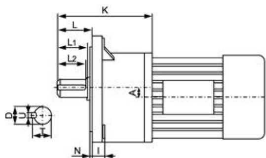
GL(H)F
