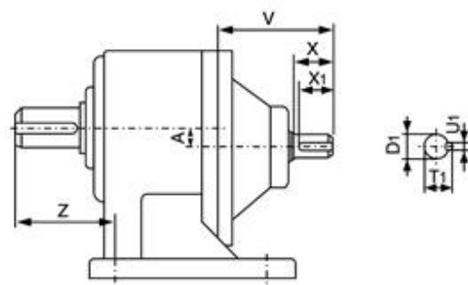
GL(H)WZ
