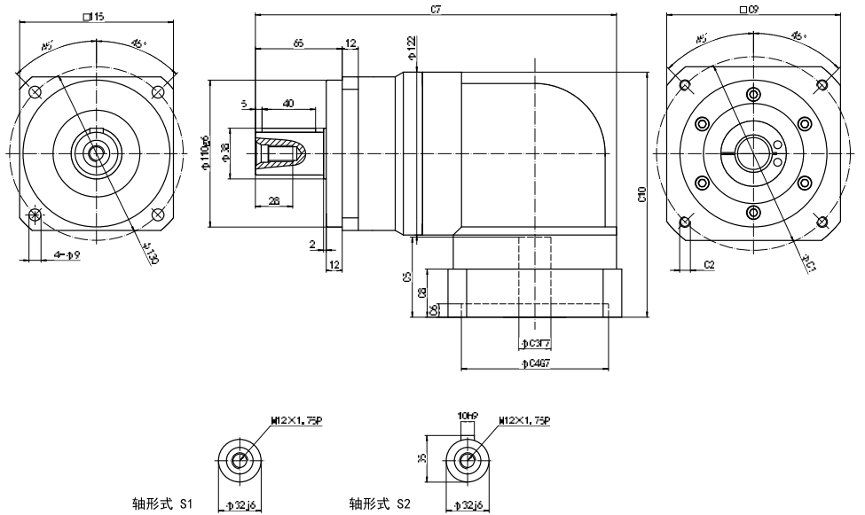
ZPFR-120-L1 外形图 Profile
