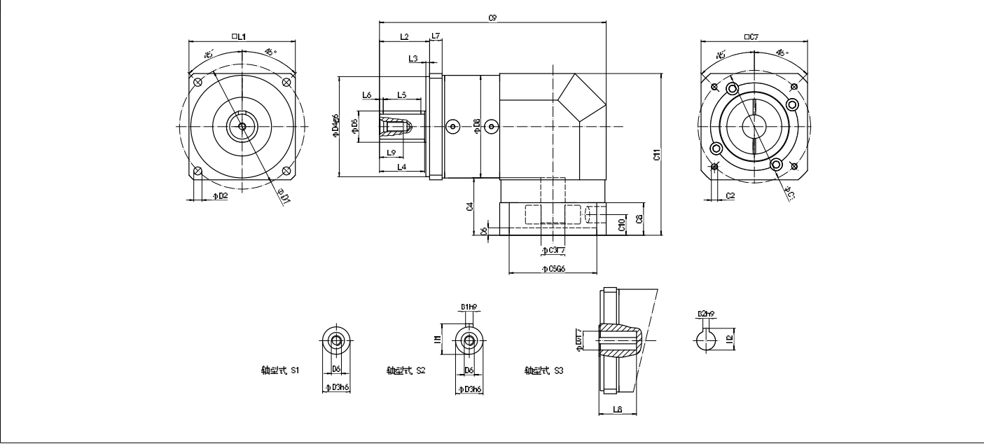
ZFR-L1 外形图 Profile
