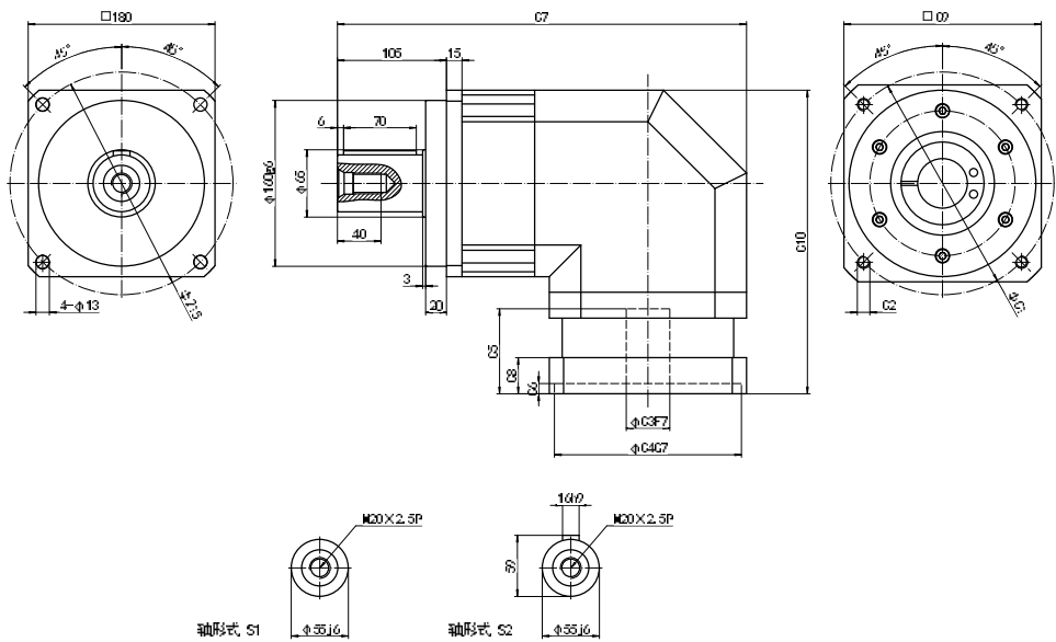
ZPBR180-L1 外形图 Profile
