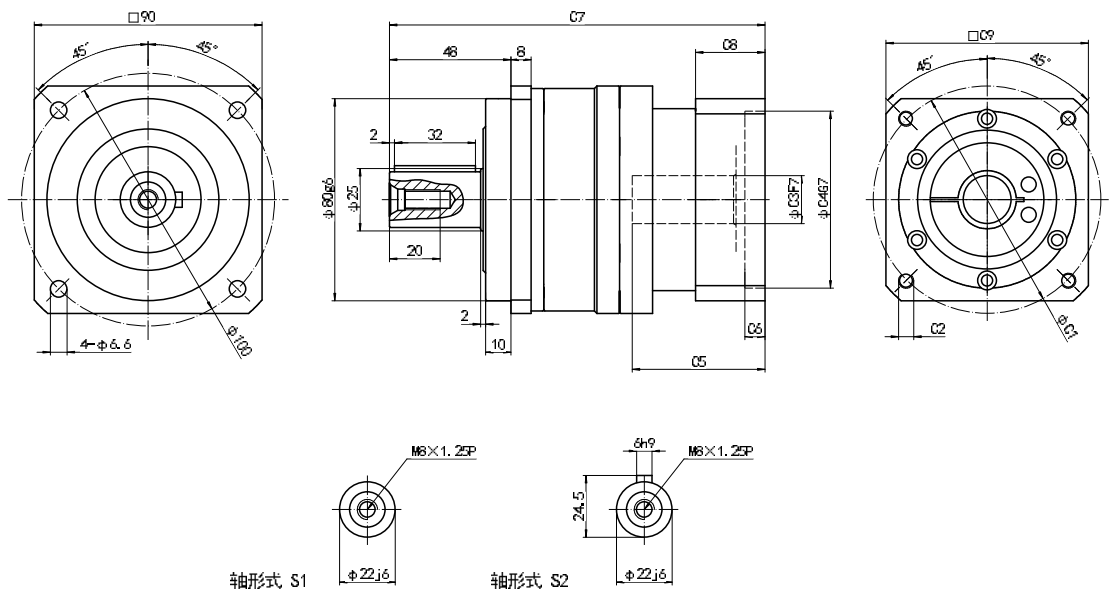
ZPF-090-L1 外形图 Profile
