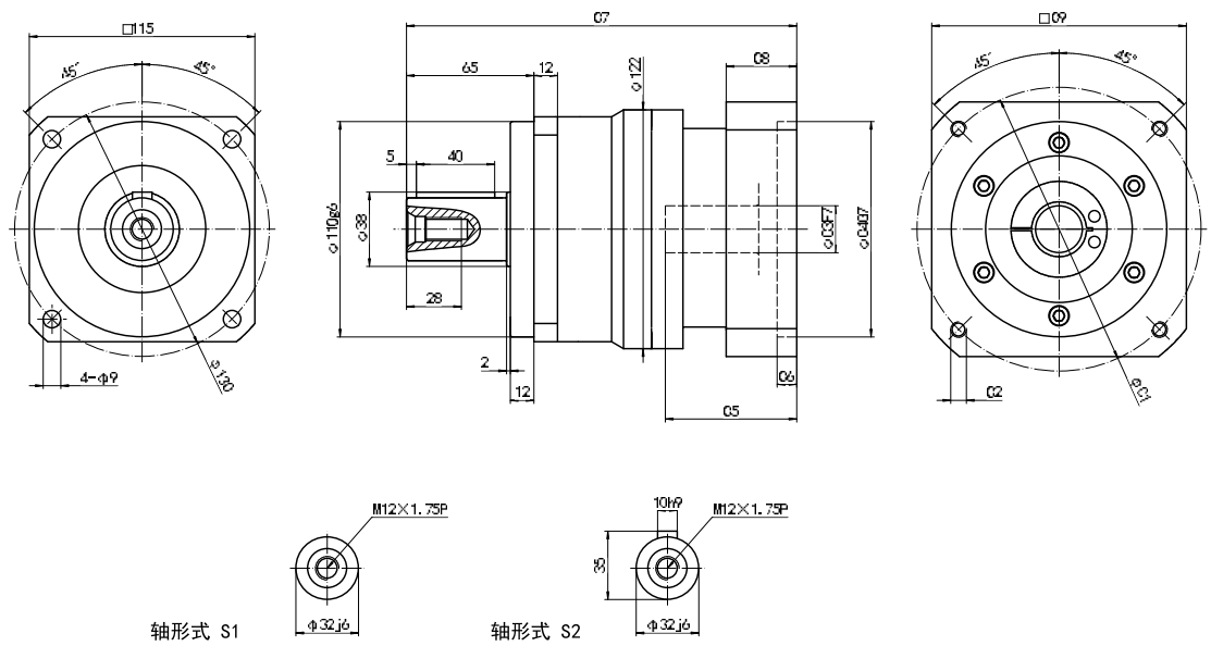
ZPF-120-L1 外形图 Profile
