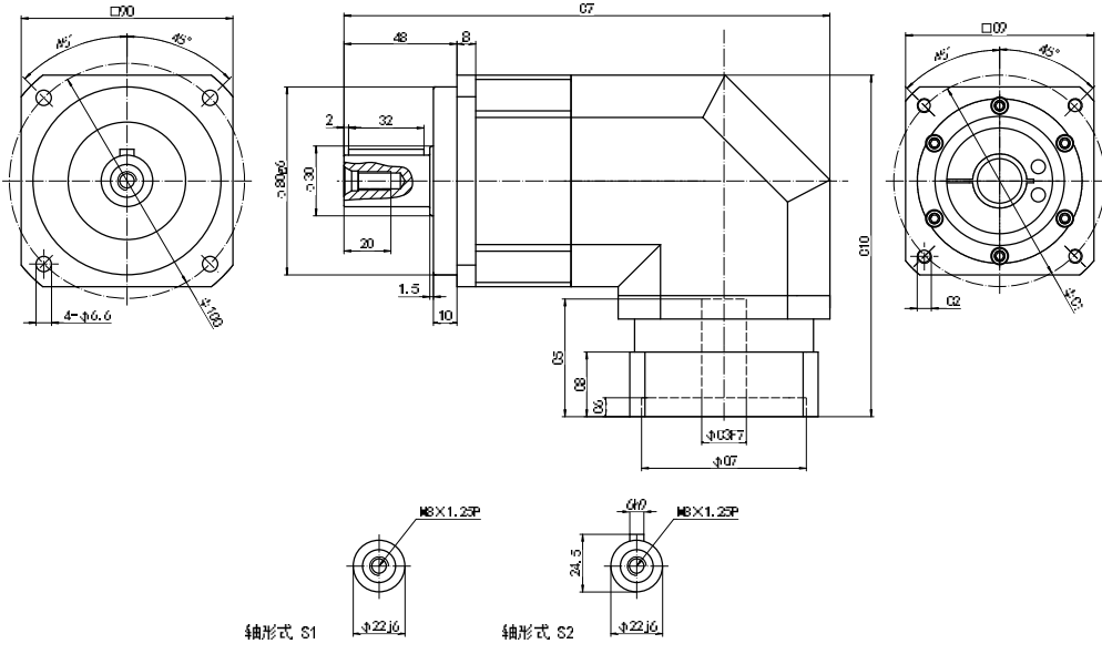
ZPBR090-L1 外形图 Profile
