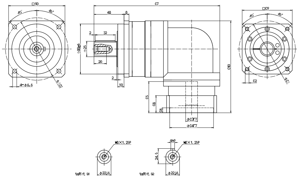
ZPFR-090-L1 外形图 Profile
