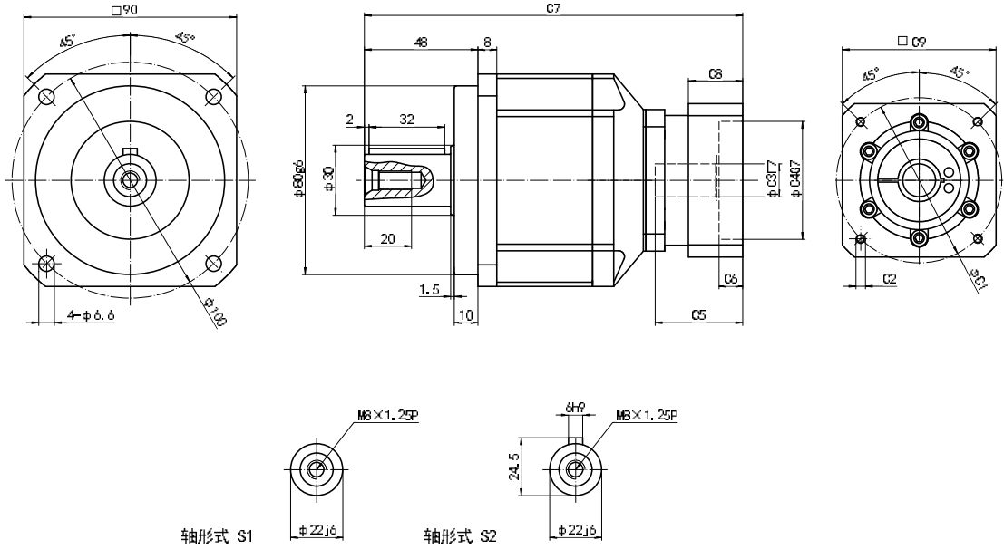
ZPB090-L2 外形图 Profile
