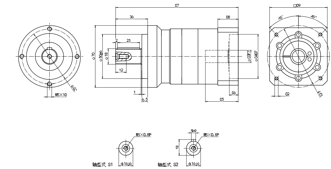
ZPE-060-L2 外形图 Profile
