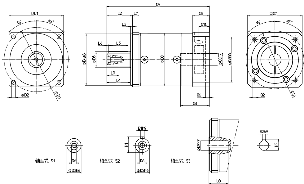
ZF-L2 外形图 Profile
