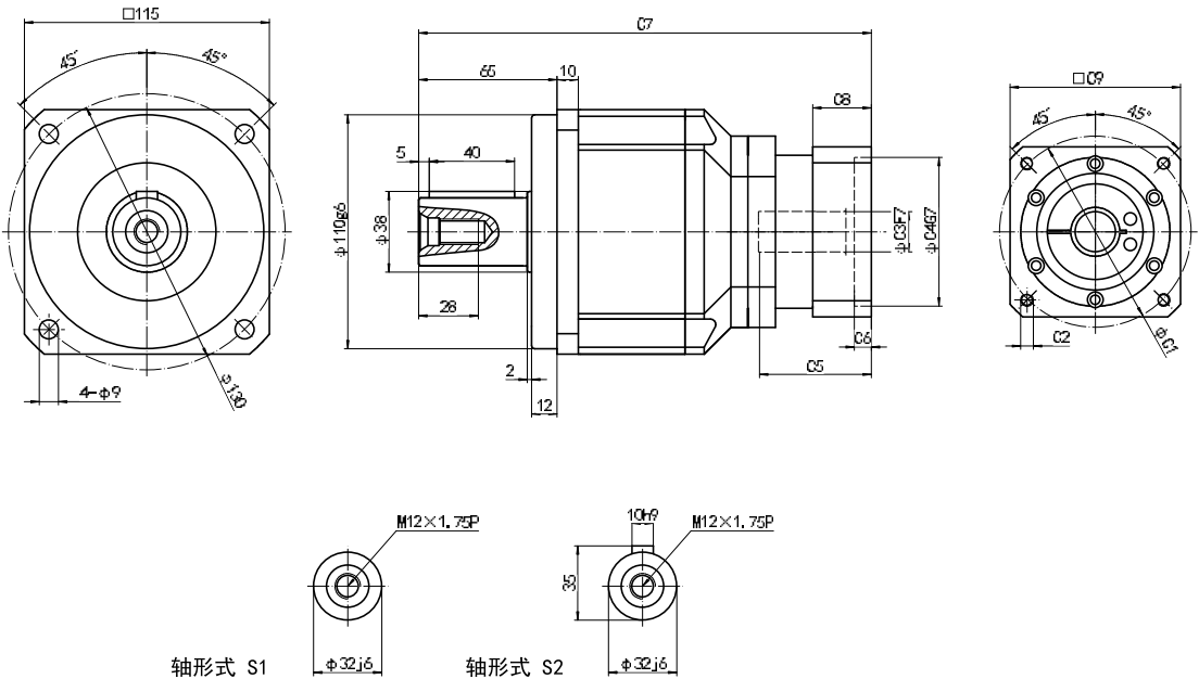
ZPB115-L2 外形图 Profile
