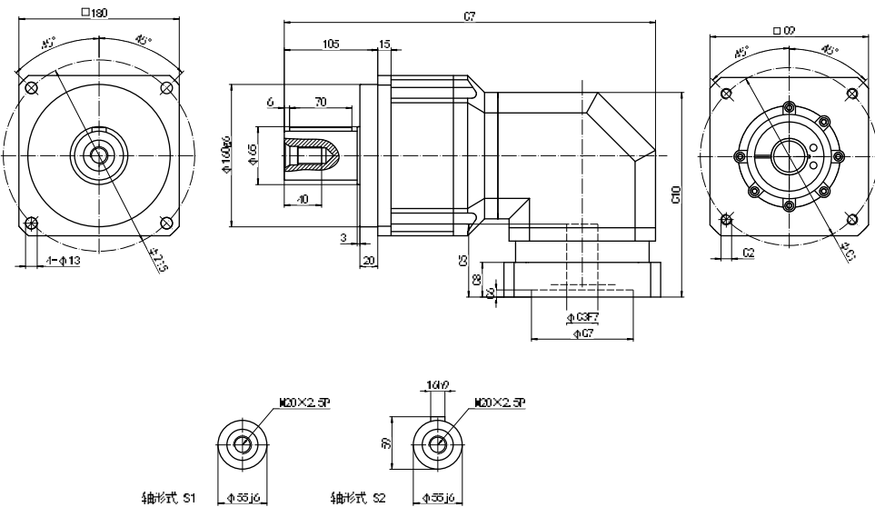
ZPBR180-L2 外形图 Profile
