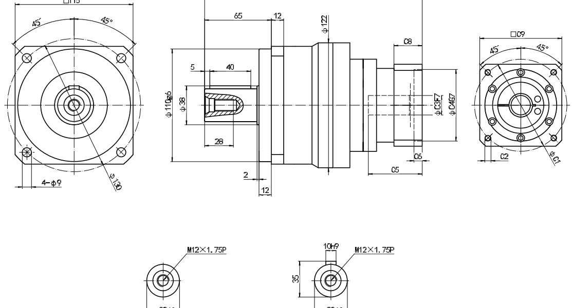
ZPF-120-L2 外形图 Profile
