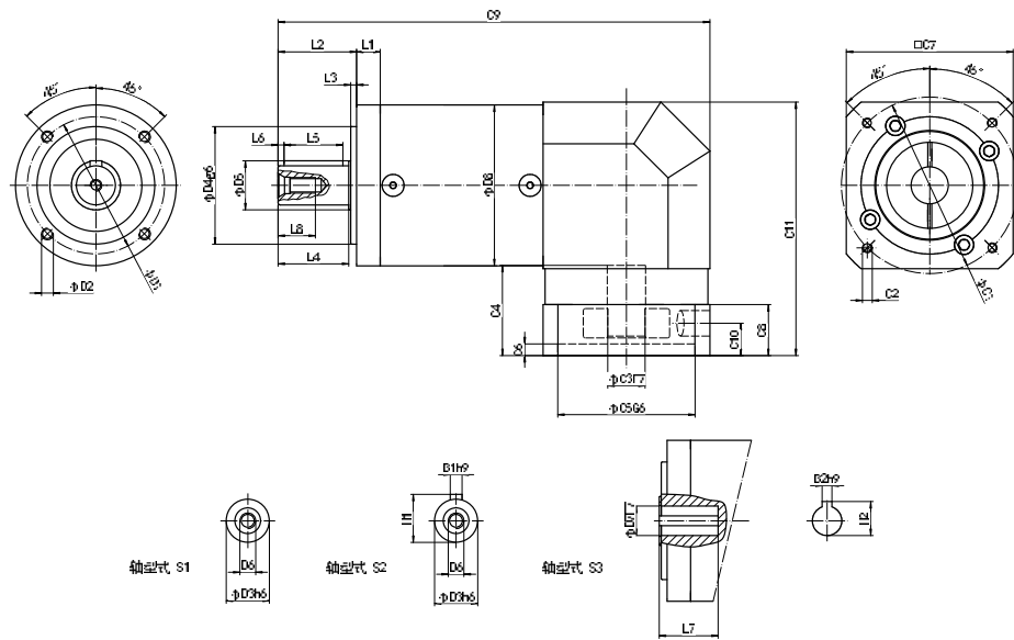
ZER-L3 外形图 Profile
