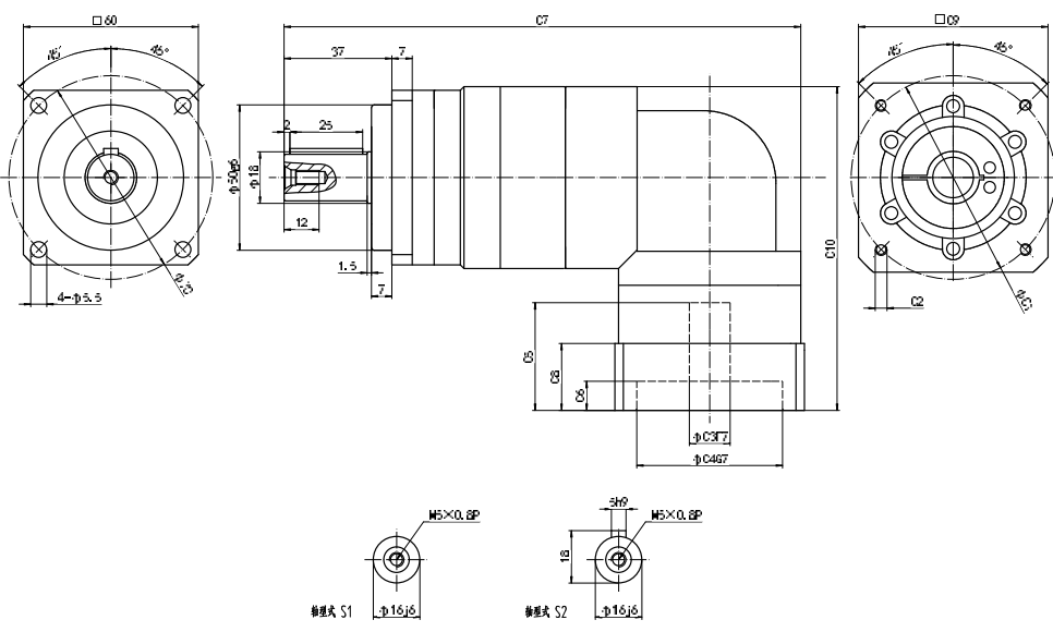
ZPFR-060-L2 外形图 Profile
