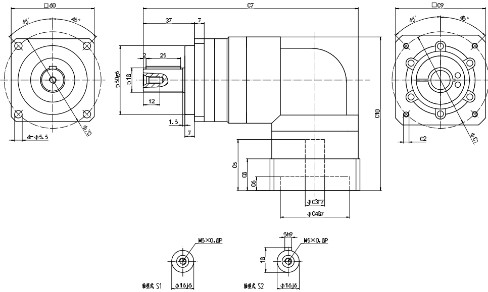
ZPFR-060-L1 外形图 Profile
