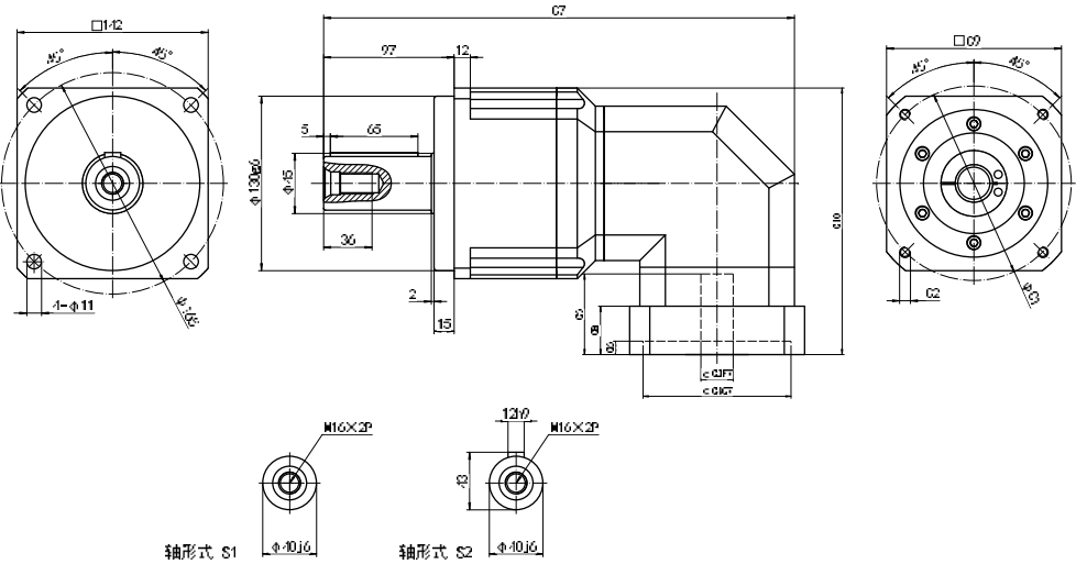
ZPBR142-L2 外形图 Profile
