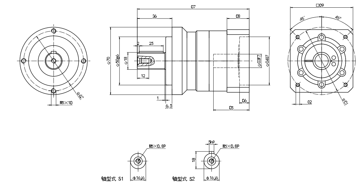
ZPE-060-L1 外形图 Profile
