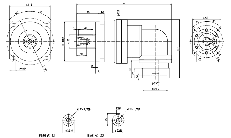
ZPFR-120-L2 外形图 Profile
