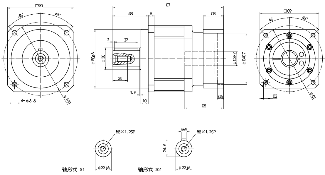
ZPB090-L1 外形图 Profile
